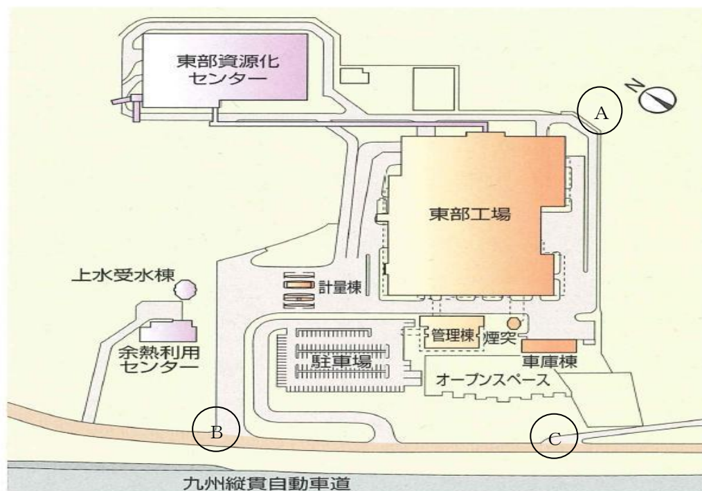
東部工場 敷地配置図
